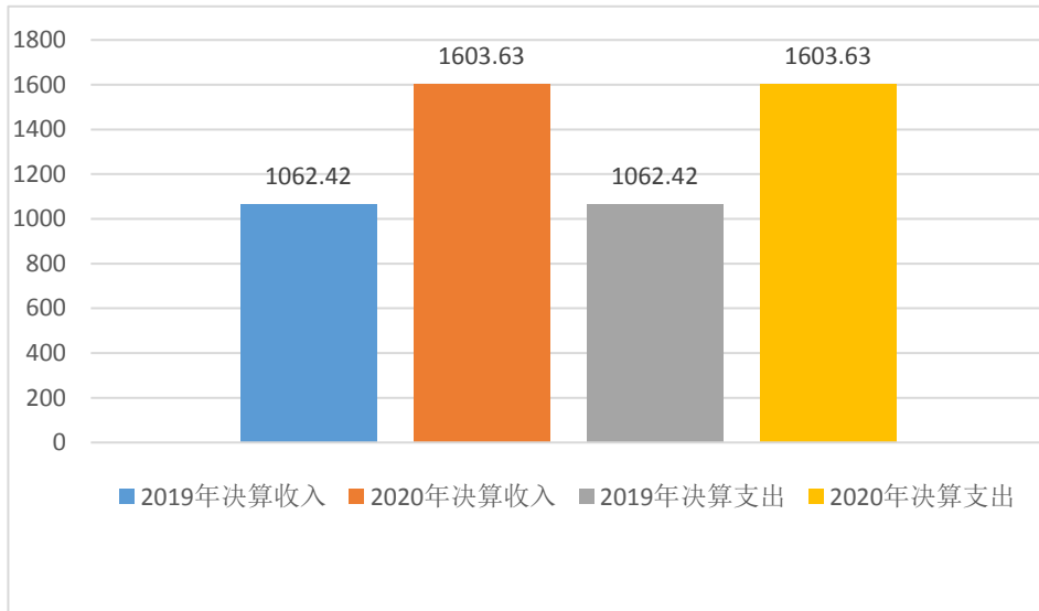
图 3: 2019-2020 年财政拨款收支对比情况
